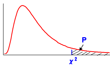
付表3 \chi^2 表
